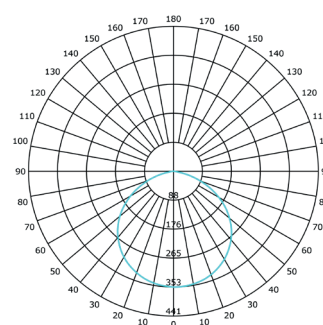
CURVA FOTOMETRICA
